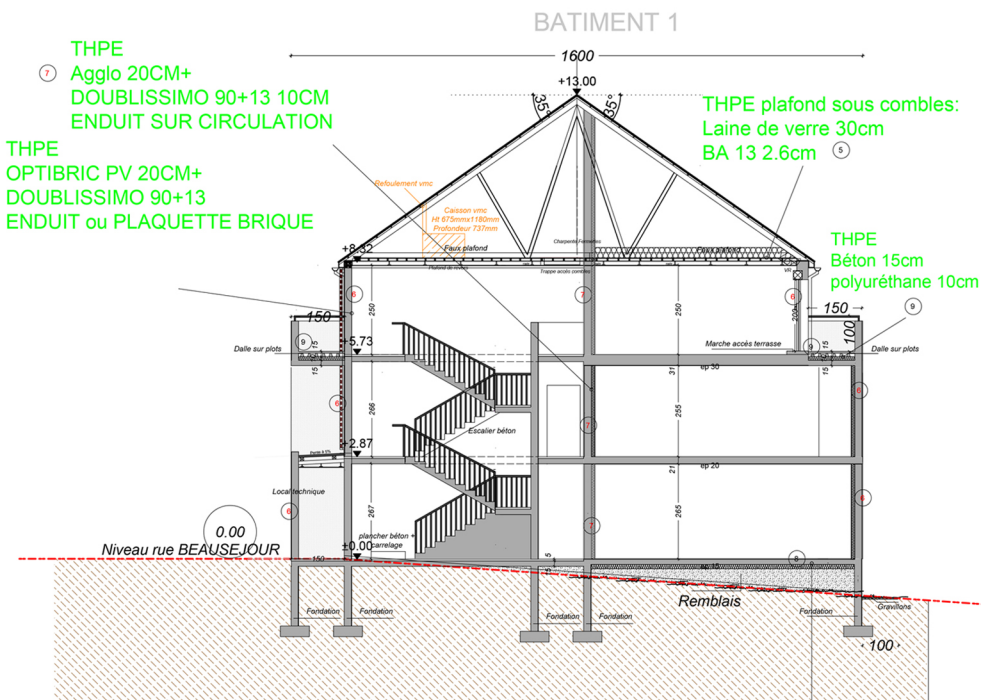
Coupe de principe AA'
