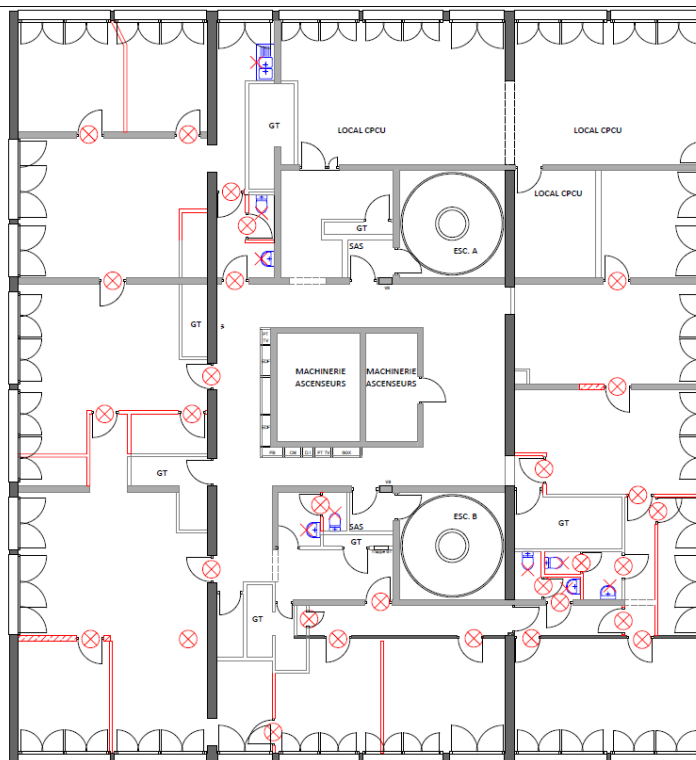
Existant - Démolition
